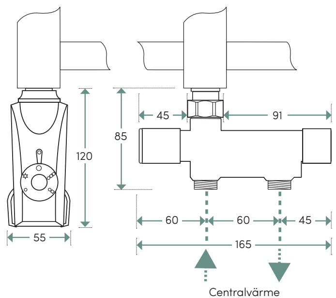
1b Alt. 1 – NH-ventil 60 c/c samt 300W elpatron*
