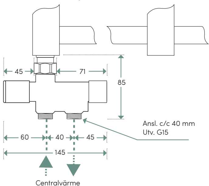
1a NH-ventil 40 C/C, manuell, anslutning neråt*
