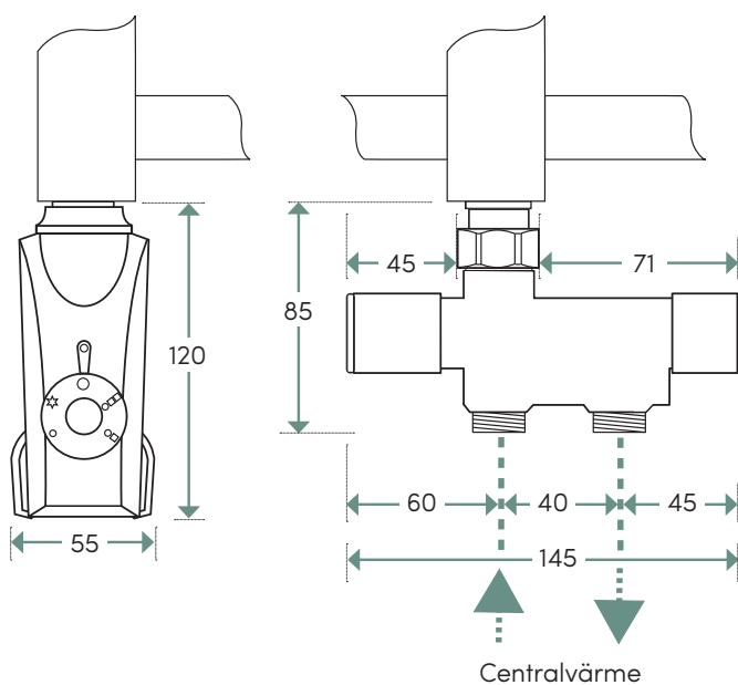
1a Alt. 1 – NH-ventil 40c/c samt 300W elpatron*
