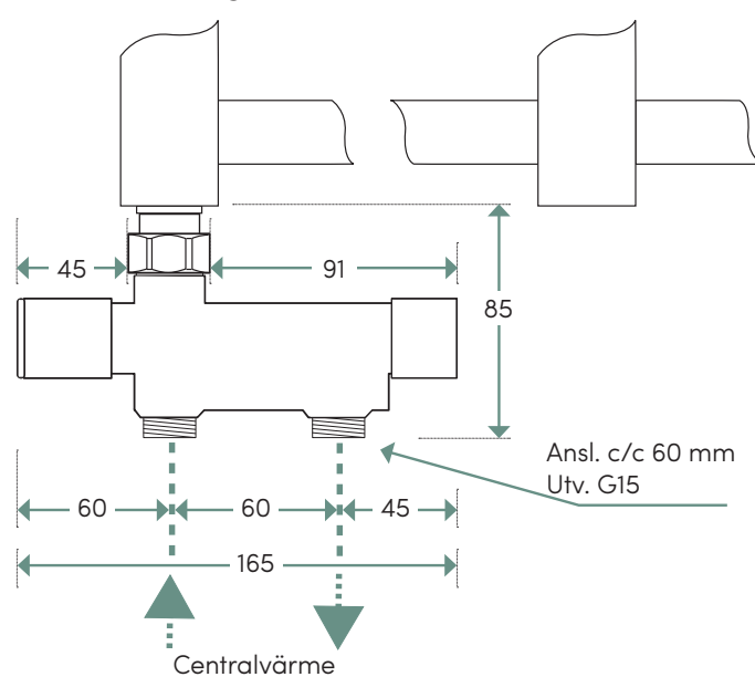
1b NH-ventil 60 C/C, manuell, anslutning neråt*
